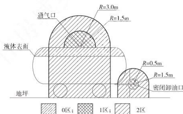
图 3-2 汽油油罐车的爆炸危险区域划分图
