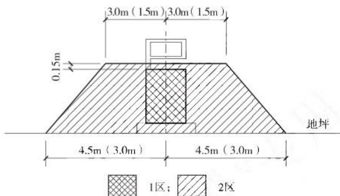
图 3-3 汽油加油机爆炸危险区域划分图
