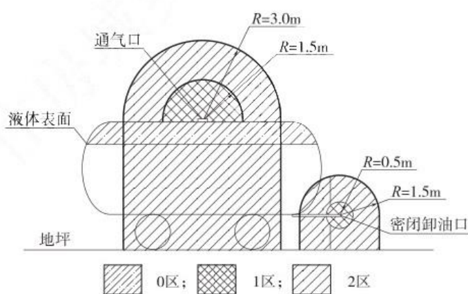
图 3-2 汽油油罐车的爆炸危险区域划分图
