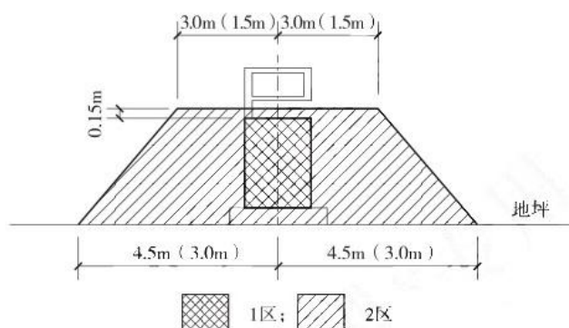
图 3-3 汽油加油机爆炸危险区域划分图
